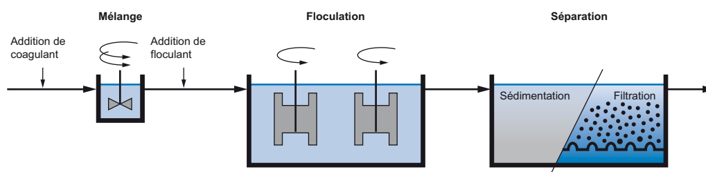
Figure 5 : Schéma d'une unité de floculation avec séparation attenante des floes (sédimentation, filtration)
